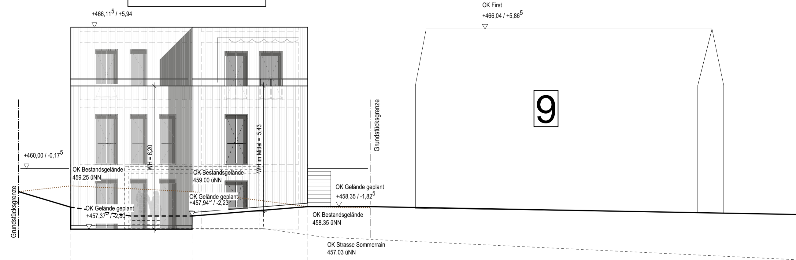
Straßenansicht Sommerrain
