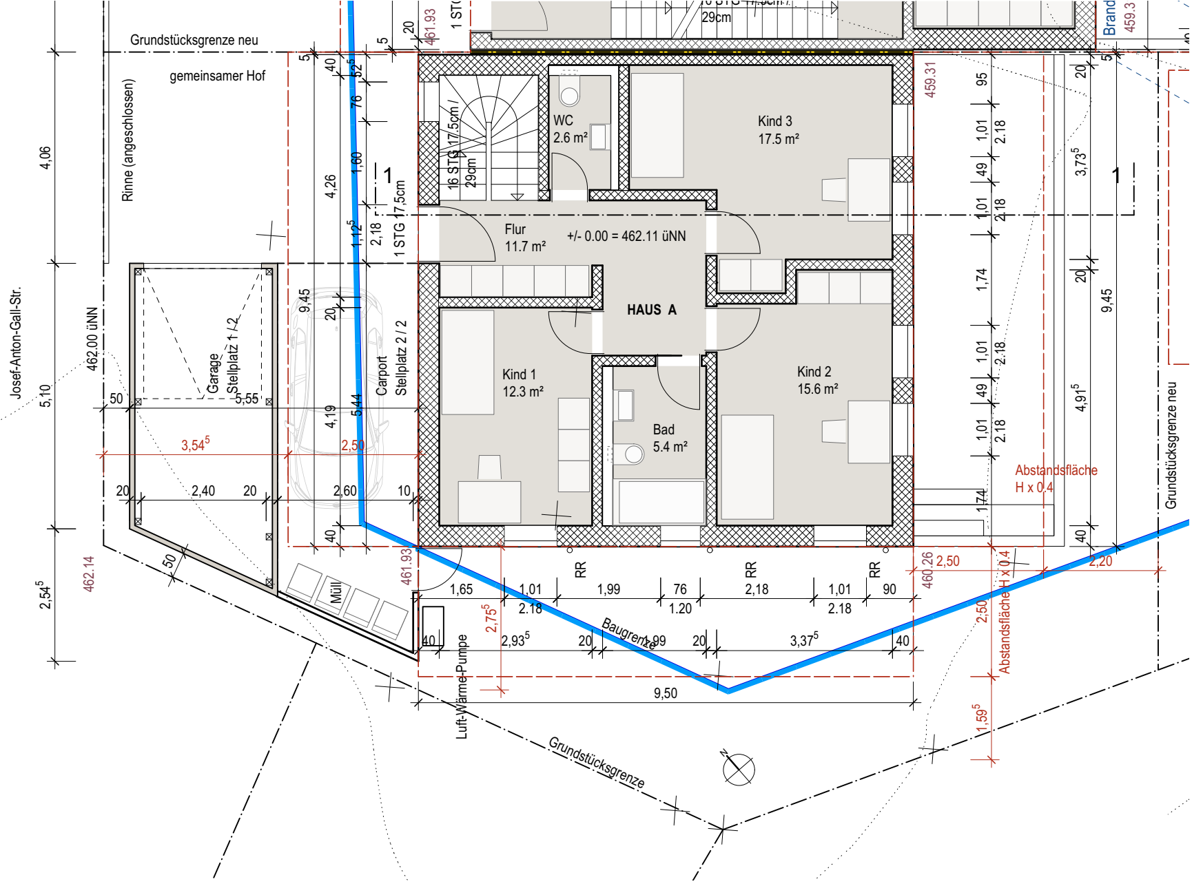
GRUNDRISS ERDGESCHOSS M 1/100
